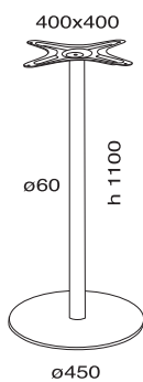
ø450 bar table base
